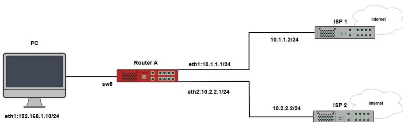
Рисунок 133 – Схема настройки IP SLA icmp
