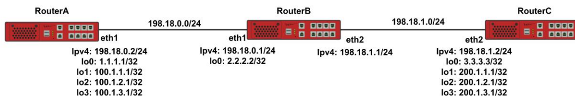
Рисунок 35 – Схема настройки фильтрации маршрутов с помощью prefix-list
