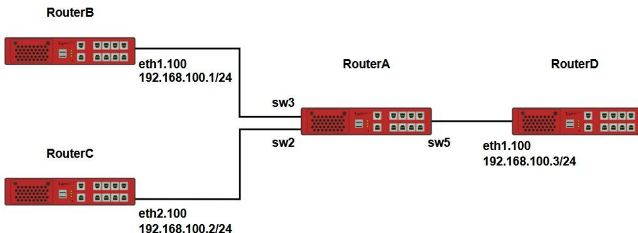
Рисунок – Схема настройки 802.1p (очередизации трафика)
