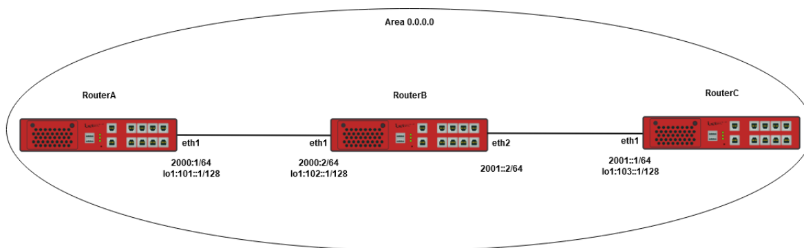
Рисунок 37 – Схема настройки протокола BFD IPv6 для динамической маршрутизации
