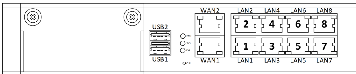
Рисунок 16 – LAN-порты. Передняя панель ISN41508T3 выпуска ранее 04.2025
