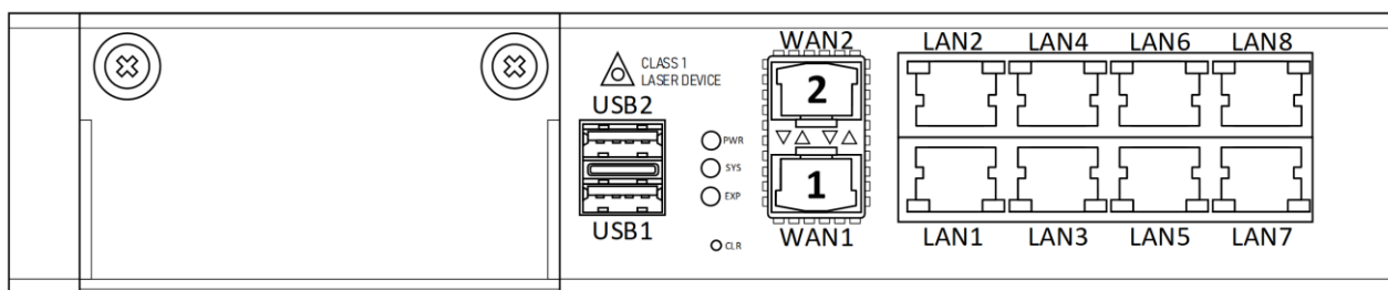
Рисунок 9 – Передняя панель ISN41508T4 выпуска ранее 04.2025
