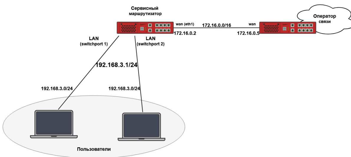
Рисунок 27 – Настройка DHCP-сервера на устройстве
