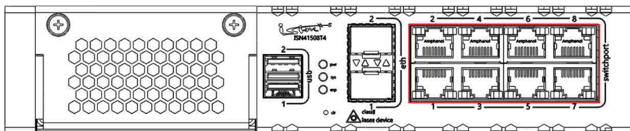
Рисунок 19 – LAN-порты. Передняя панель ISN41508T4
