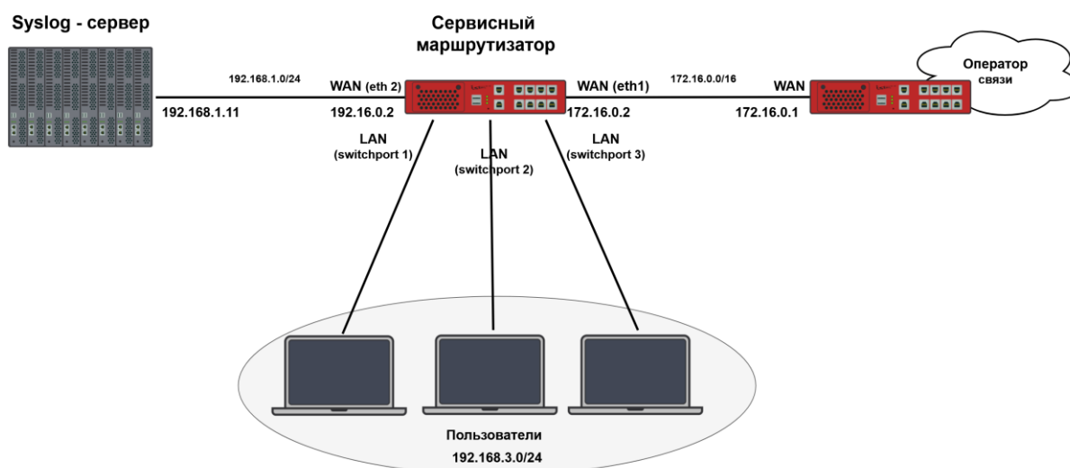
Рисунок 28 – Схема настройки журналирования событий на удаленный Syslog-сервер
