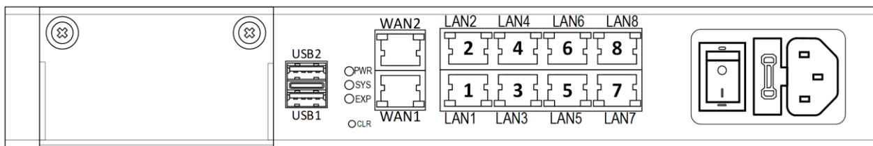
Рисунок 22 – LAN-порты. Передняя панель ISN41508T3-M-AC выпуска ранее 04.2025
