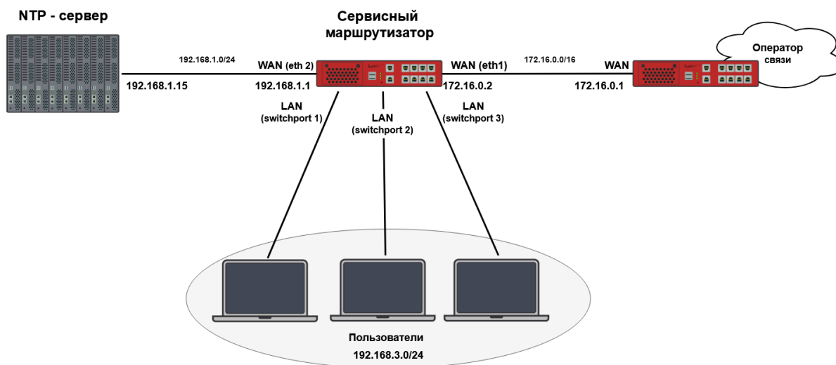
Рисунок 29 – Настройка синхронизации времени с NTP-сервера
