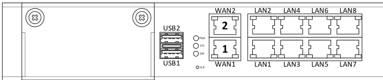
Рисунок 7 – Передняя панель ISN41508T3-M выпуска ранее 04.2025
