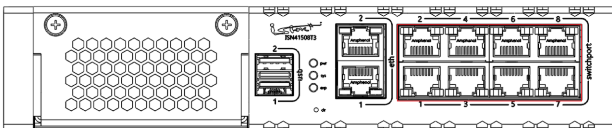
Рисунок 15 – LAN-порты. Передняя панель ISN41508T3
