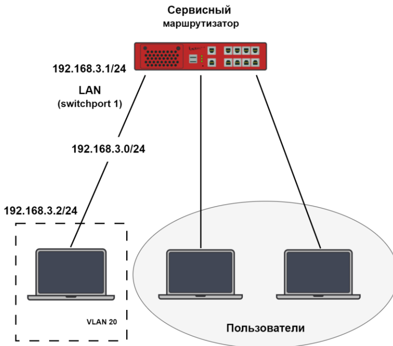
Рисунок 23 – Схема настройки локальной сети
