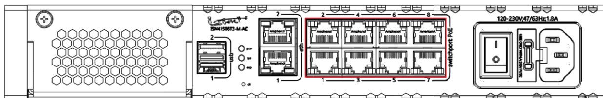
Рисунок 21 – LAN-порты. Передняя панель ISN41508T3-M-AC
