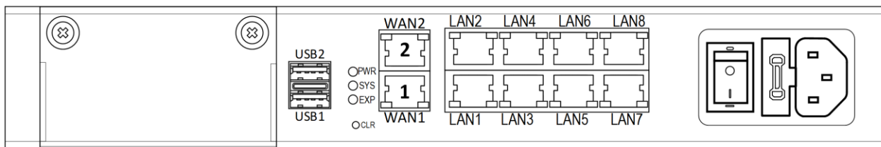
Рисунок 11 – Передняя панель ISN41508T3-M-AC выпуска ранее 04.2025
