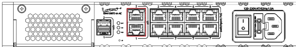
Рисунок 10 – Передняя панель ISN41508T3-M-AC
