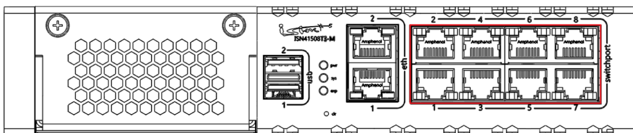
Рисунок 17 – LAN-порты. Передняя панель ISN41508T3-M
