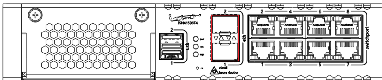
Рисунок 8 – Панель передняя ISN41508T4
