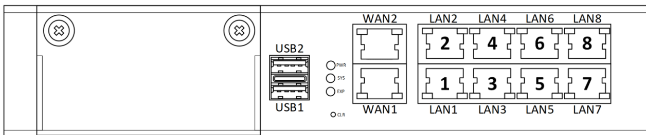
Рисунок 18 – LAN-порты. Передняя панель ISN41508T3-M выпуска ранее 04.2025
