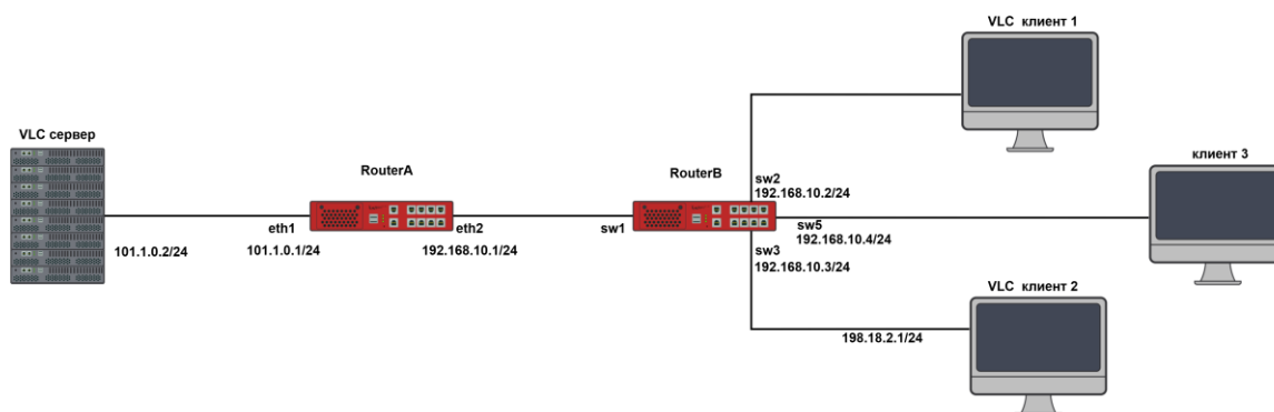
Рисунок 68 – Схема настройки IGMP snooping
