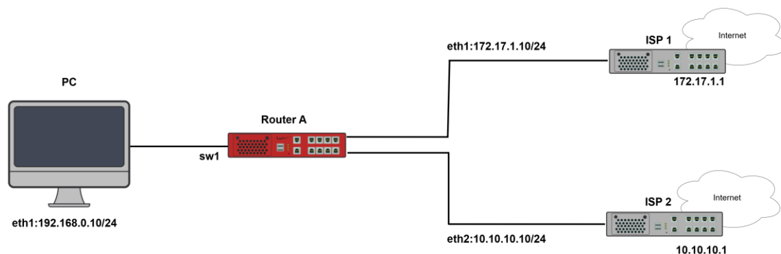
Рисунок 132 – Схема настройки IP SLA
