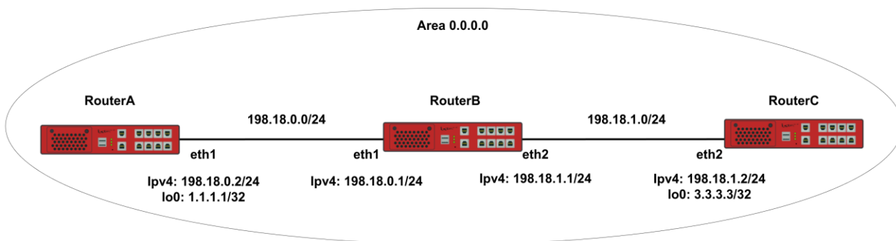
Рисунок 36 – Схема настройки протокола BFD для динамической маршрутизации
