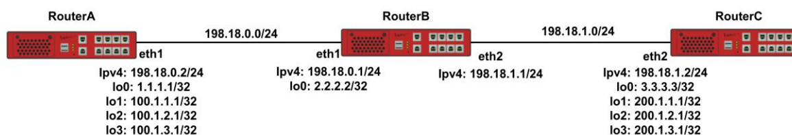
Рисунок 35 – Схема настройки фильтрации маршрутов с помощью prefix-list
