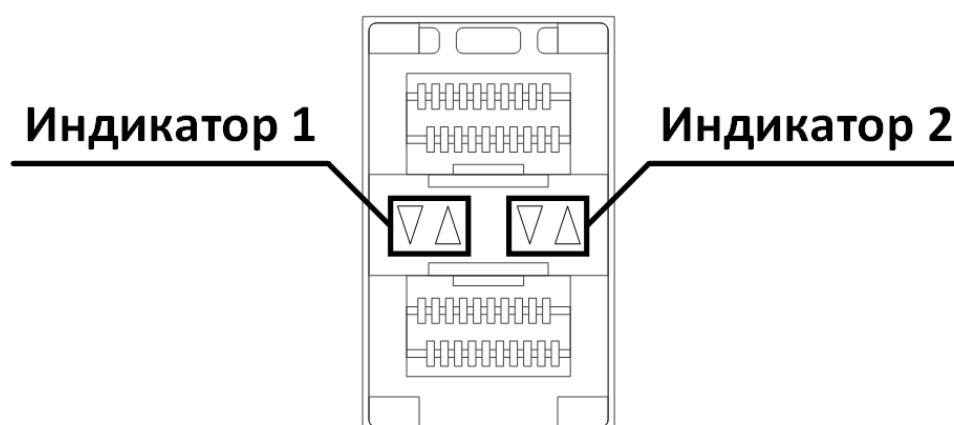
Рисунок 30 – Индикаторы состояния SFP-интерфейсов
