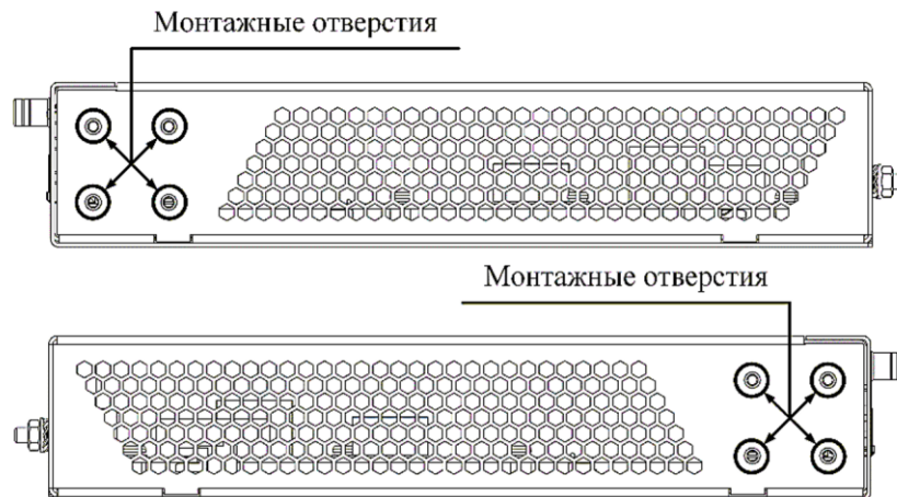
Рисунок 31 – Монтажные отверстия изделия
