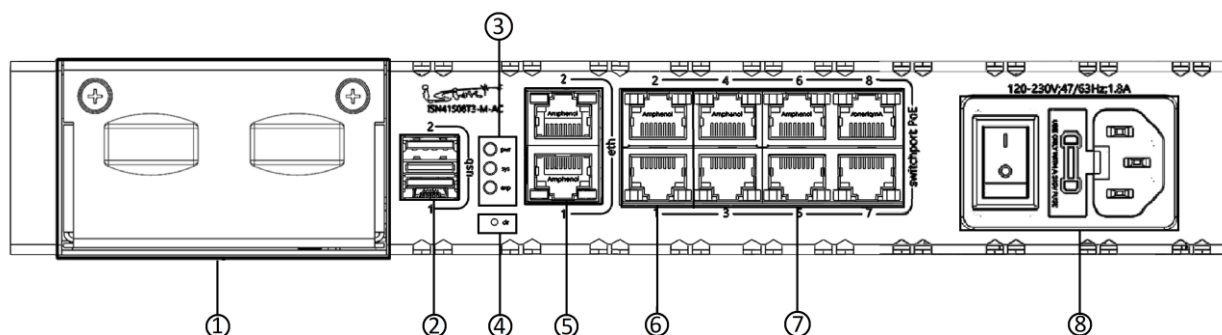
Рисунок 24 – Конфигурация элементов передней панели изделия
