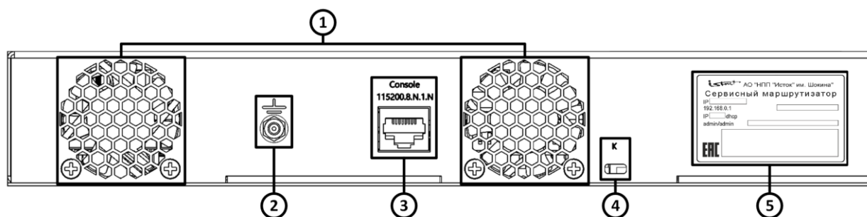
Рисунок 10 – Конфигурация элементов задней панели изделия ISN41508T3-M-AC
