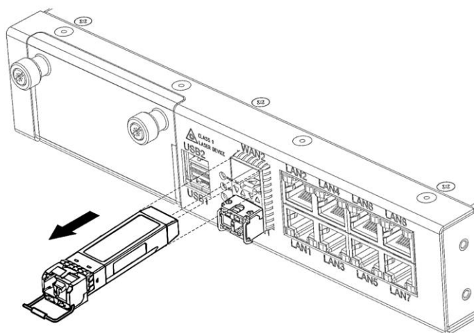
Рисунок 43 – Извлечение SFP-трансивера из слота
