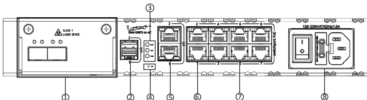
Рисунок 22 – Конфигурация элементов передней панели изделия ISN41508T3-M-AC/ISES0116
