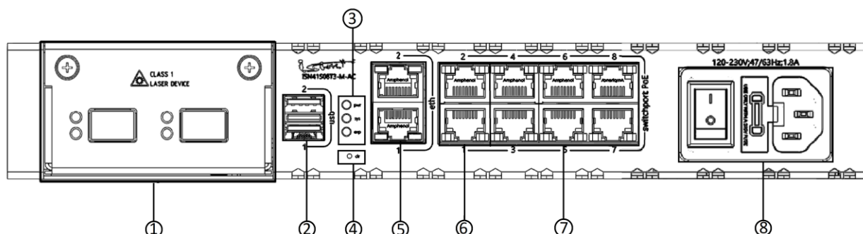
Рисунок 18 – Конфигурация элементов передней панели изделия ISN41508T3-M-AC/ISES1004
