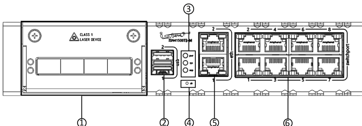
Рисунок 14 – Конфигурация элементов передней панели изделия ISN41508T3-M/ISES0108
