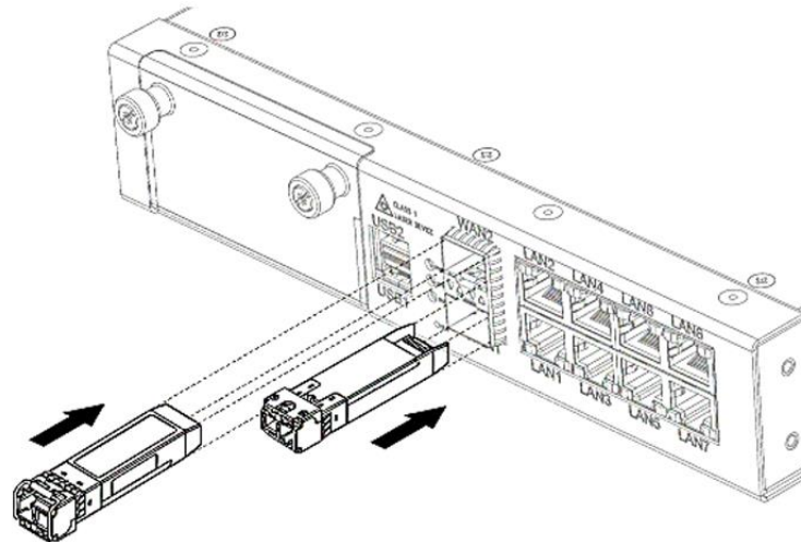
Рисунок 38 – Установка SFP-трансиверов в слоты изделия
