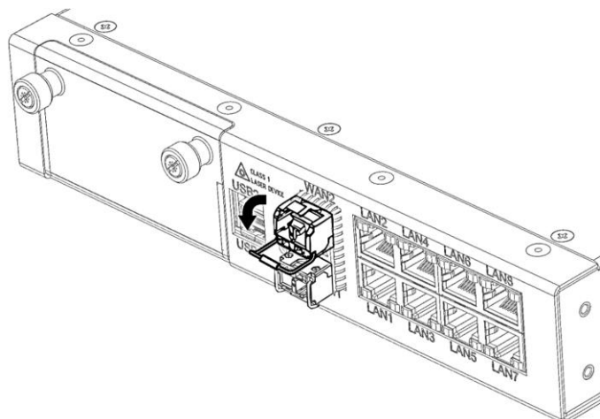
Рисунок 42 – Разблокирование удерживающей защелки
