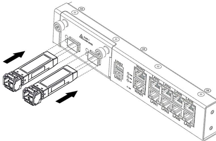
Рисунок 39 – Установка SFP-трансиверов в слоты модулей расширения
