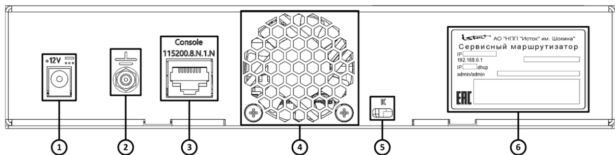
Рисунок 3 – Конфигурация элементов задней панели изделия ISN41508T3
