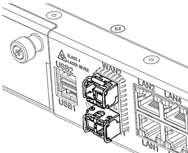
Рисунок 40 – SFP-трансиверы, установленные в слоты изделия
