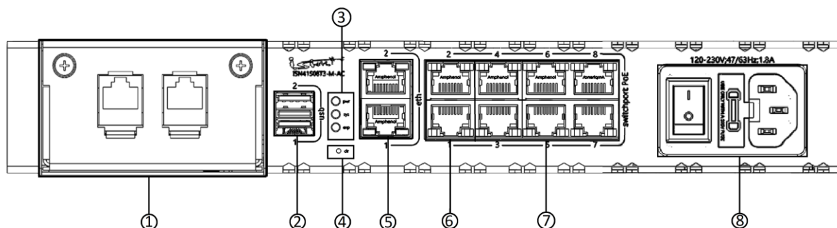
Рисунок 26 – Конфигурация элементов передней панели изделия
