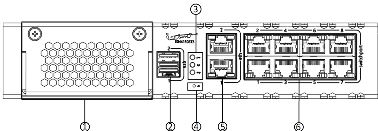
Рисунок 2 – Конфигурация элементов передней панели изделия ISN41508T3
