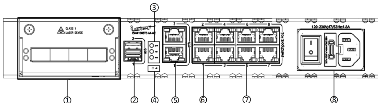
Рисунок 20 – Конфигурация элементов передней панели изделия ISN41508T3-M-AC/ISES0108
