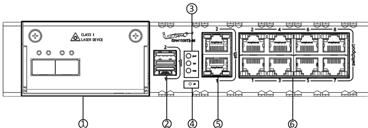
Рисунок 16 – Конфигурация элементов передней панели изделия ISN41508T3-M/ISES0116
