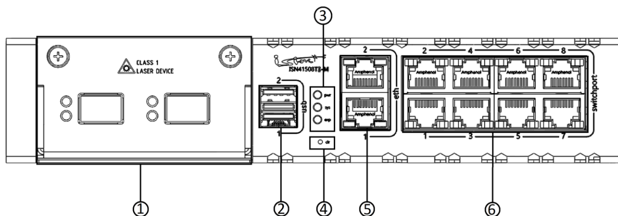
Рисунок 12 – Конфигурация элементов передней панели изделия ISN41508T3-M/ISES1004
