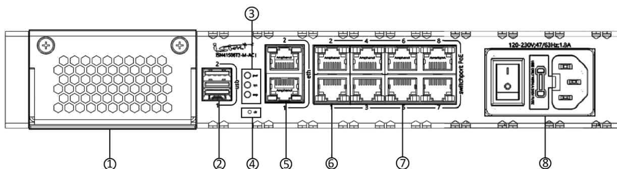
Рисунок 9 – Конфигурация элементов передней панели изделия ISN41508T3-M-AC
