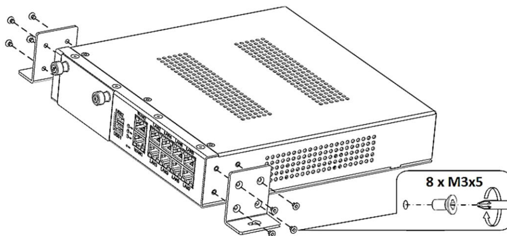
Рисунок 36 – Крепление уголков из комплекта КРПГ.465961.002
