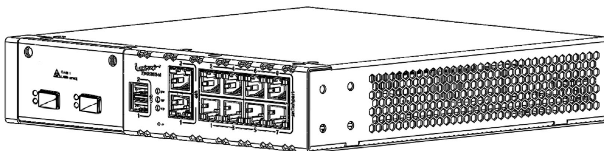
Рисунок 11 – Общий вид изделия ISN41508T3-M/ISES1004
