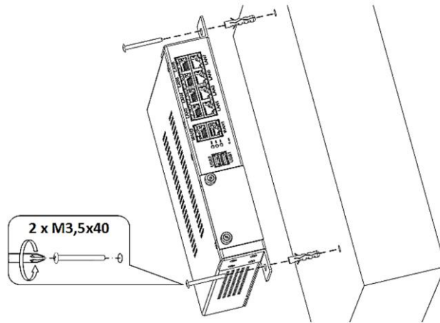
Рисунок 37 – Крепление изделий к стене с использованием комплекта КРПГ.465961.002
