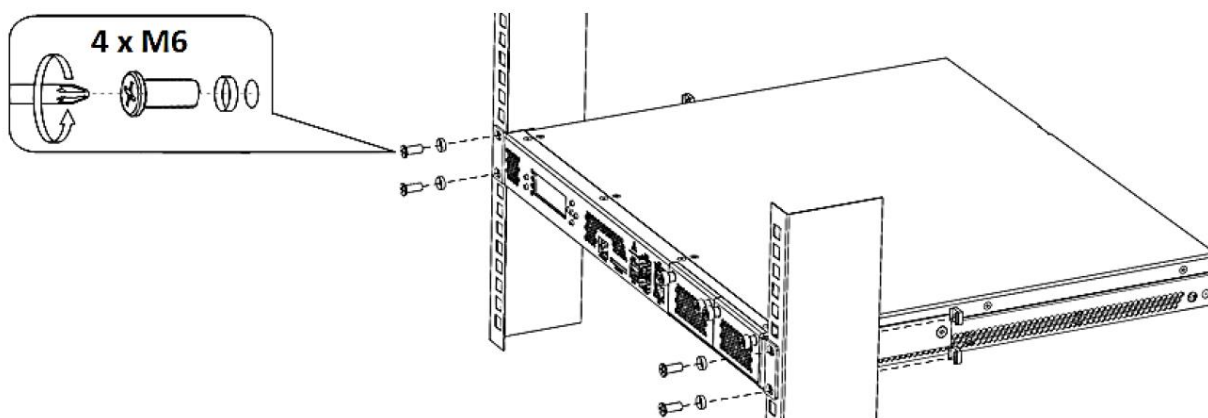
Рисунок 24 – Установка изделий в стойку с использованием комплекта КРПГ.465961.008
