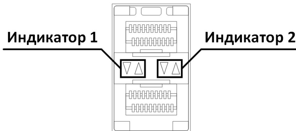
Рисунок 21 – Индикаторы состояния SFP-интерфейсов
