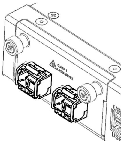
Рисунок 28 – SFP-трансиверы, установленные в слоты модуля расширения
