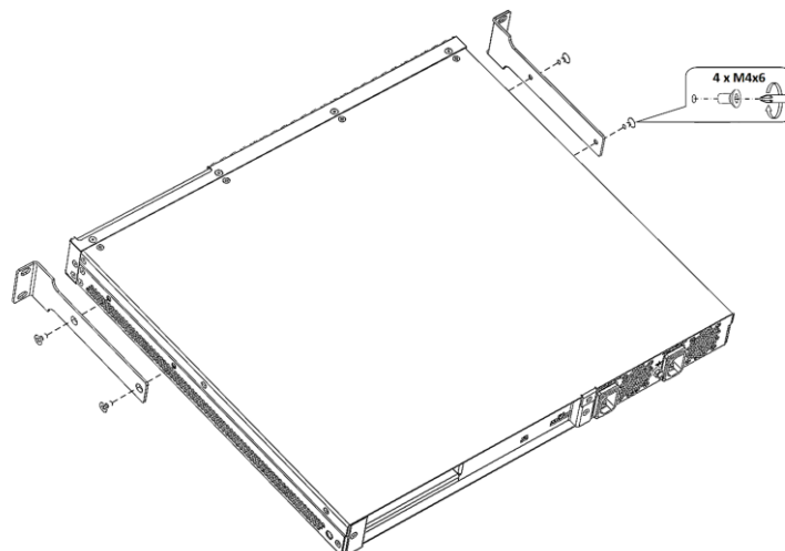
Рисунок 23 – Крепление кронштейнов из комплекта для монтажа в стойку КРПГ.465961.008
