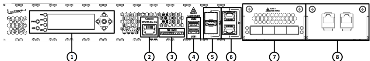
Рисунок 8 – Конфигурация элементов передней панели изделия ISN50502T5-M13A
