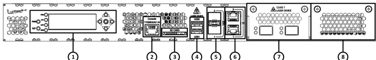
Рисунок 12 – Конфигурация элементов передней панели изделия ISN50502T5-M15A
