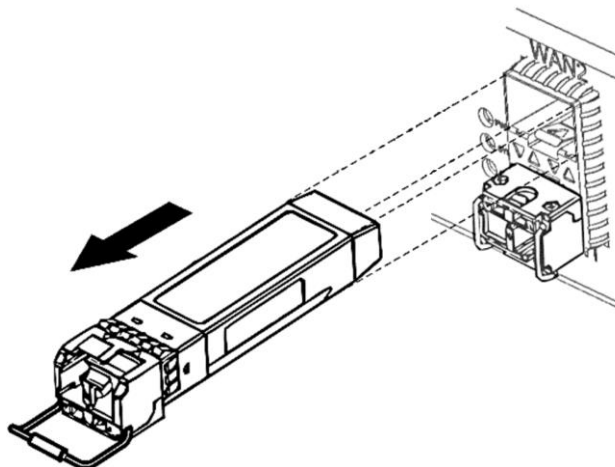
Рисунок 30 – Извлечение SFP-трансивера из слота
