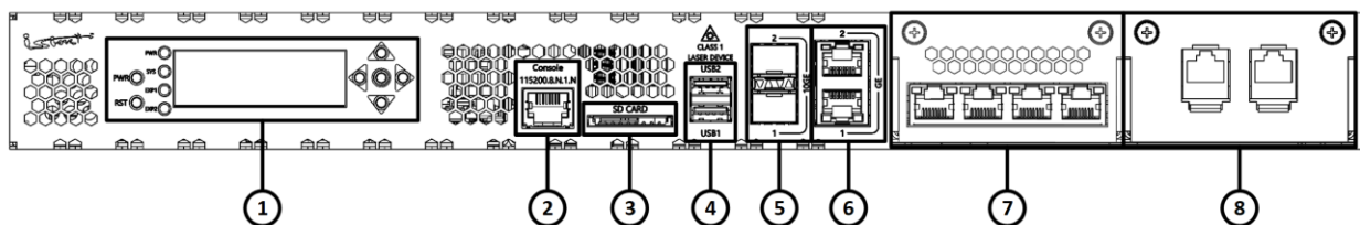
Рисунок 4 – Конфигурация элементов передней панели изделия ISN50502T5-M11A
