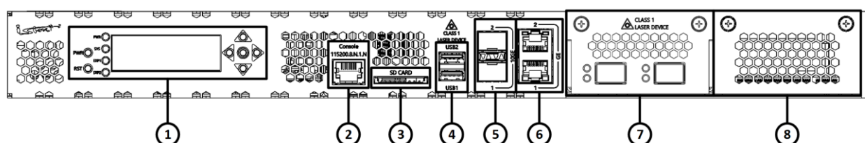
Рисунок 10 – Конфигурация элементов передней панели изделия ISN50502T5-M14A
