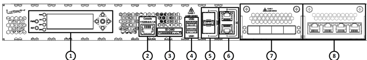
Рисунок 19 – Конфигурация элементов передней панели изделия
