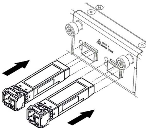
Рисунок 26 – Установка SFP-трансиверов в слоты модулей расширения
