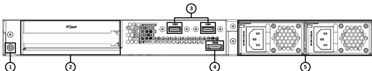
Рисунок 17 – Конфигурация элементов задней панели изделия
