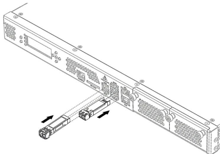
Рисунок 25 – Установка SFP-трансиверов в слоты изделия
