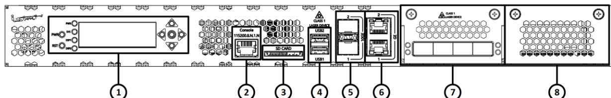
Рисунок 14 – Конфигурация элементов передней панели изделия ISN50502T5-M16A
