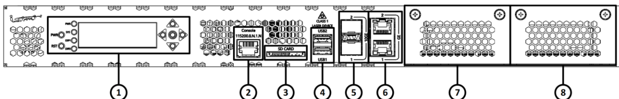
Рисунок 16 – Конфигурация элементов передней панели
