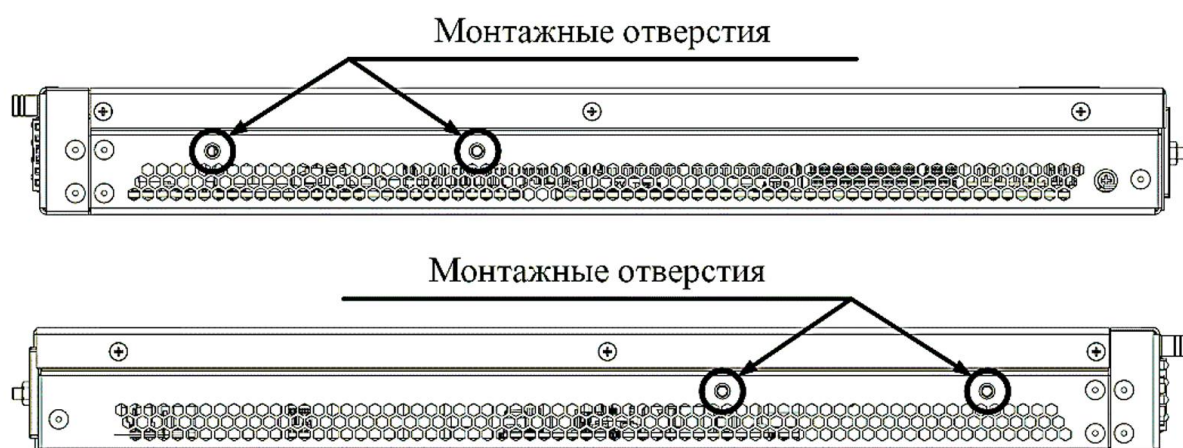
Рисунок 22 – Монтажные отверстия изделия
