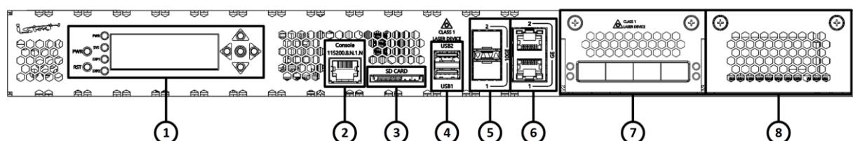
Рисунок 6 – Конфигурация элементов передней панели изделия ISN50502T5-M12A
