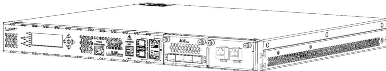
Рисунок 7 – Общий вид изделия ISN50502T5-M13A
