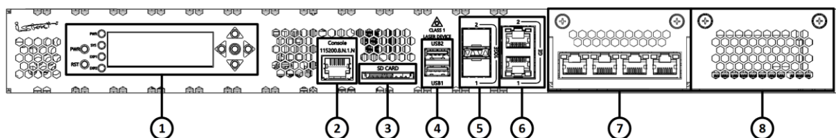
Рисунок 2 – Конфигурация элементов передней панели изделия ISN50502T5-M10A
