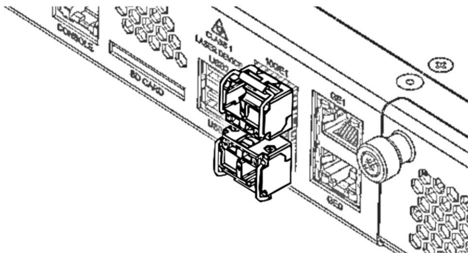
Рисунок 27 – SFP-трансиверы, установленные в слоты изделия
