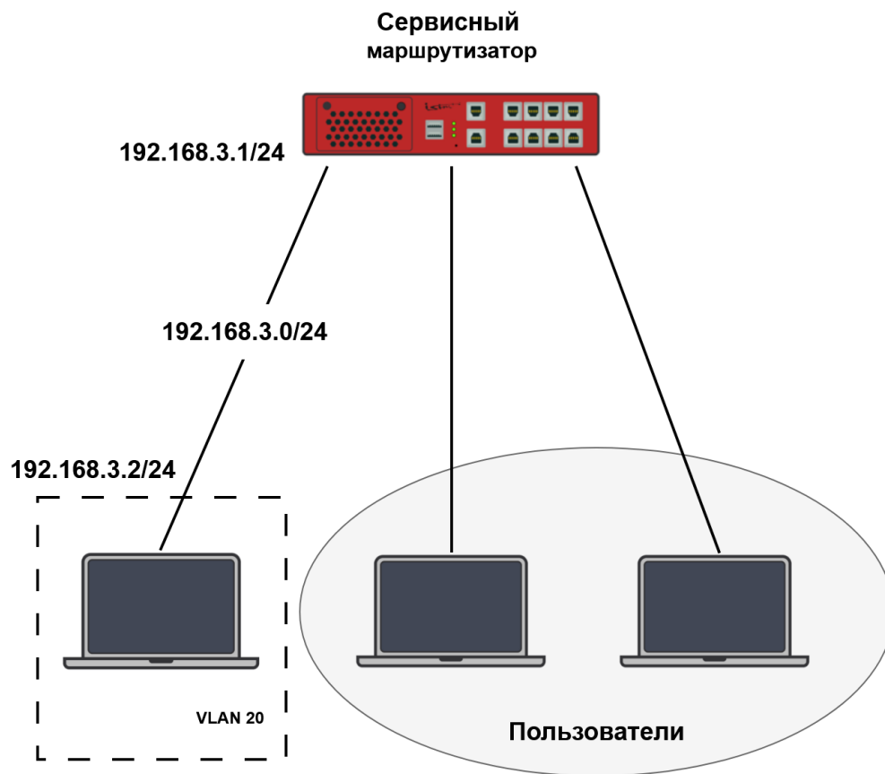
Рисунок 7 – Схема настройки локальной сети
