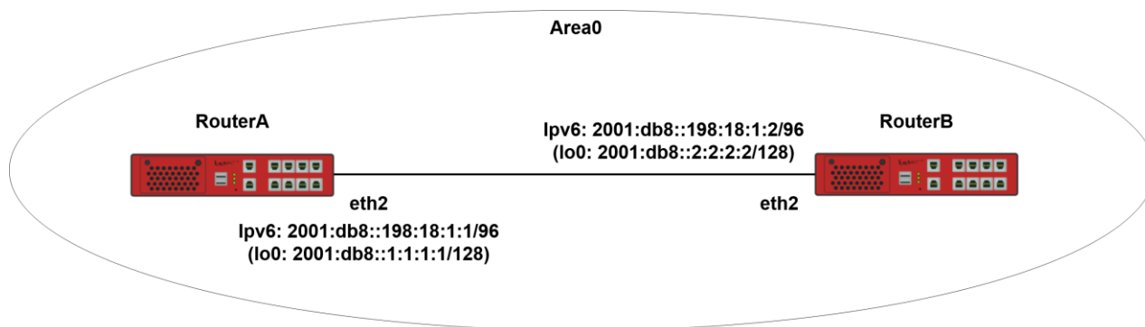
Рисунок 24 – Схема настройки динамической маршрутизации OSPFv3
