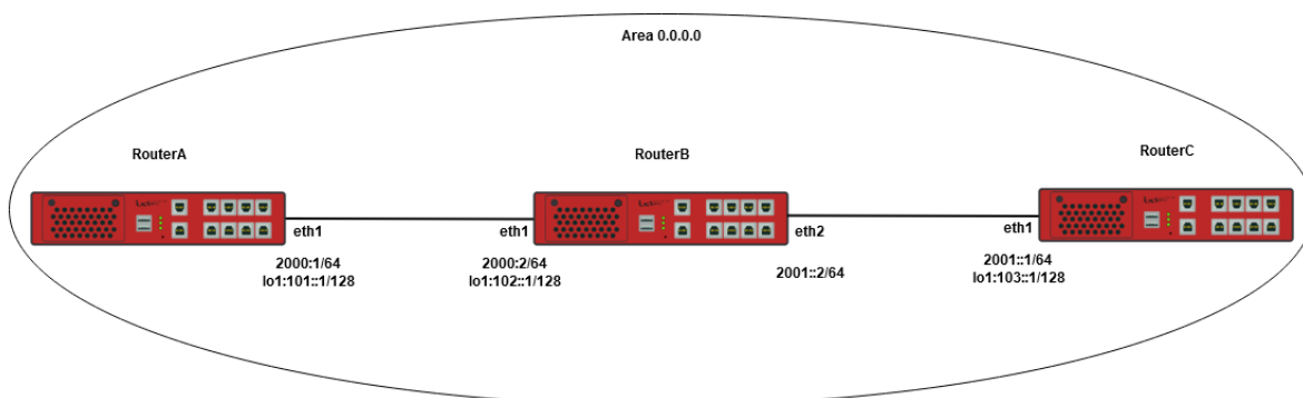
Рисунок 30 – Схема настройки протокола BFD IPv6 для динамической маршрутизации
