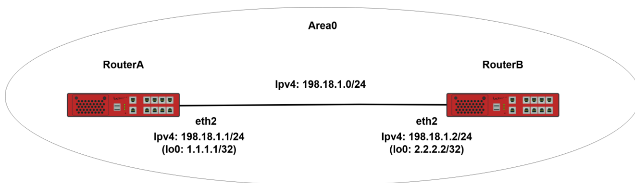
Рисунок 23 – Схема настройки динамической маршрутизации OSPFv2
