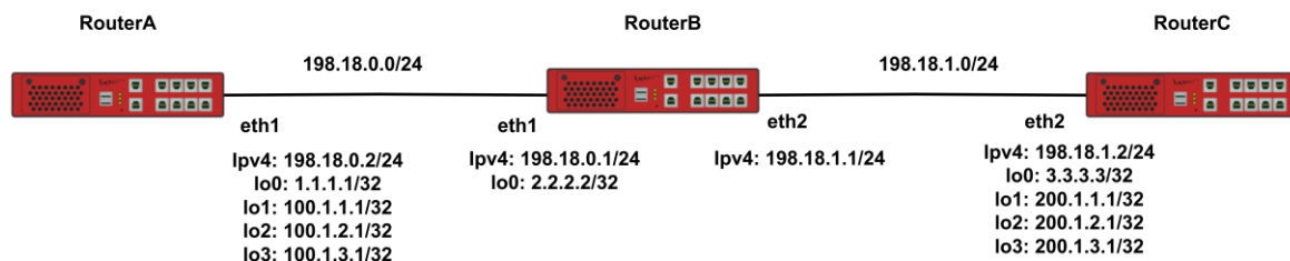
Рисунок 26 – Схема настройки протокола динамической маршрутизации BGP
