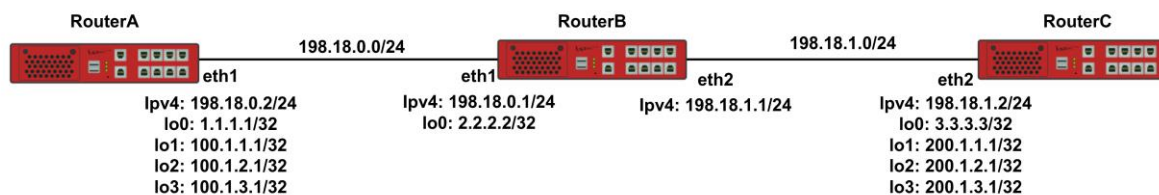
Рисунок 28 – Схема настройки фильтрации маршрутов с помощью prefix-list
