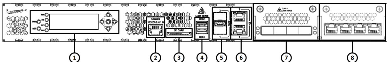
Рисунок 19 – Конфигурация элементов передней панели изделия
