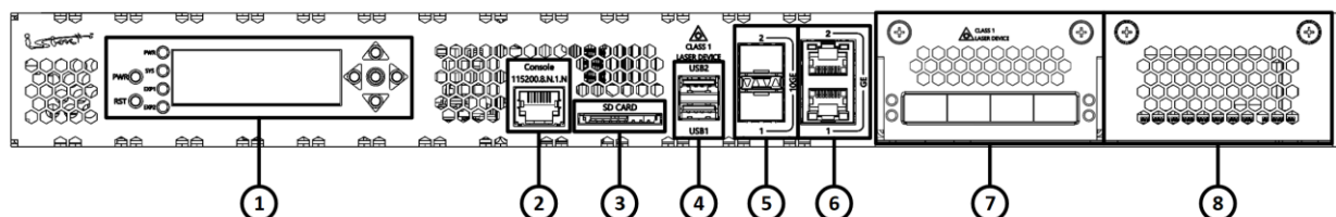
Рисунок 14 – Конфигурация элементов передней панели изделия ISN50502T5-M16A
