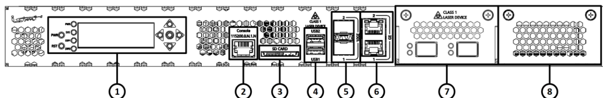
Рисунок 12 – Конфигурация элементов передней панели изделия ISN50502T5-M15A
