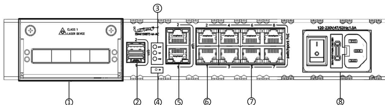
Рисунок 20 – Конфигурация элементов передней панели изделия ISN41508T3-M-AC/ISES0108
