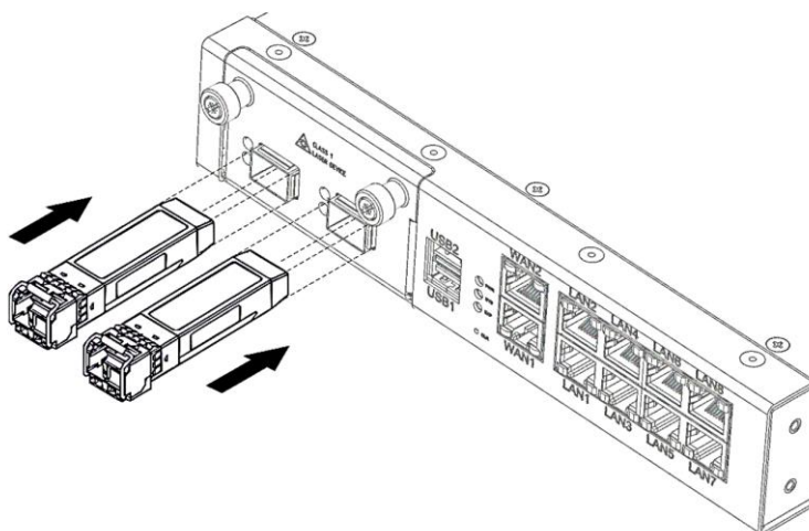
Рисунок 39 – Установка SFP-трансиверов в слоты модулей расширения
