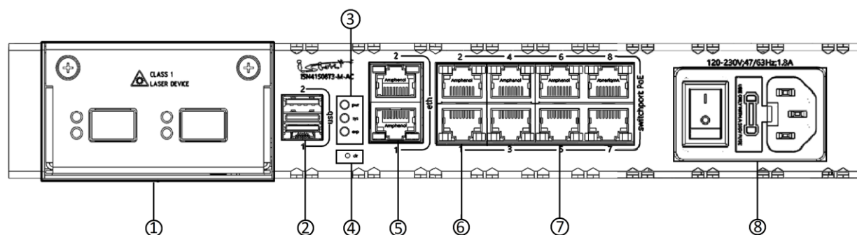
Рисунок 18 – Конфигурация элементов передней панели изделия ISN41508T3-M-AC/ISES1004
