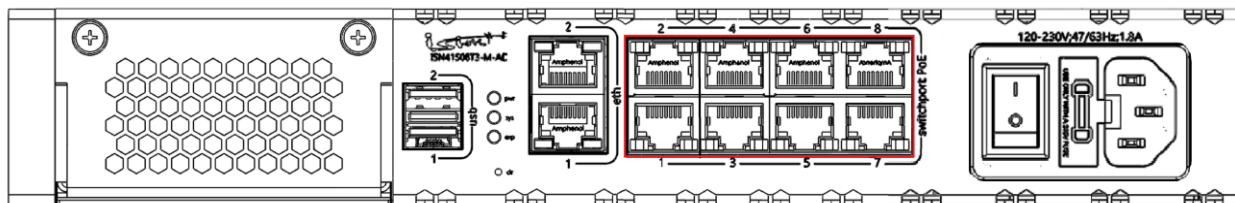
Рисунок 14 – LAN-порты. Передняя панель ISN41508T3-M-AC
