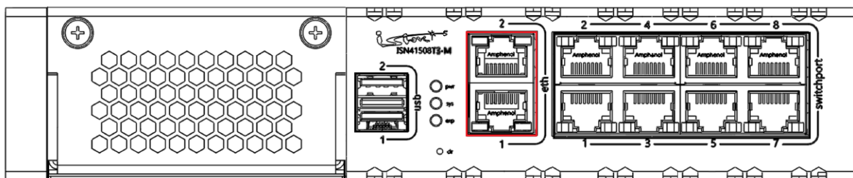
Рисунок 5 – Передняя панель ISN41508T3-M
