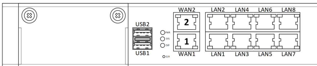
Рисунок 4 – WAN-порты. Передняя панель ISN41508T3
