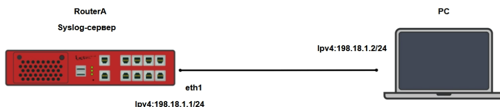
Рисунок 108 – Схема настройки сервера Syslog
