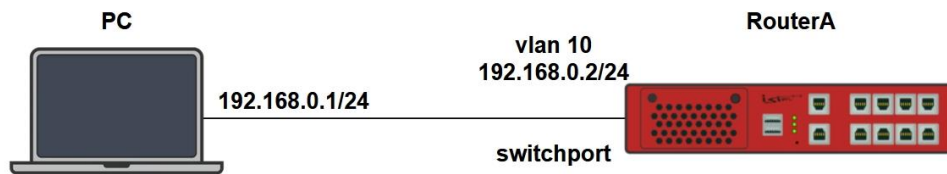
Рисунок 15 – Схема настройки VLAN
