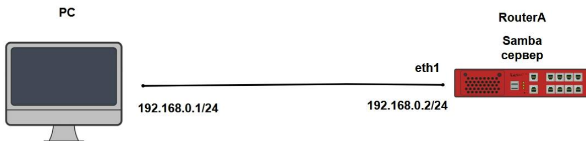
Рисунок 117 – Схема настройки работы сервера Samba
