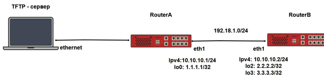
Рисунок 51 – Схема настройки loopback-интерфейса в качестве next-hop для статического маршрута
