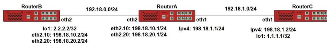
Рисунок 48 – Схема настройки PBR на основе номера порта назначения
