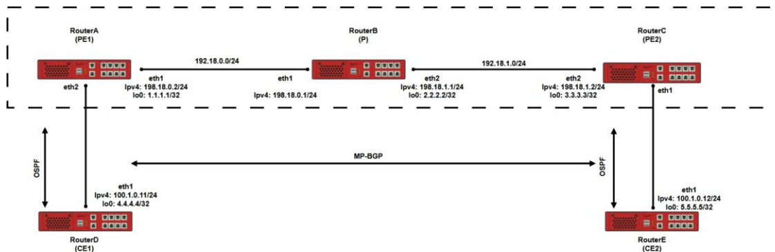
Рисунок 65 – Создание виртуальных частных сетей третьего уровня (MPLS L3VPN)
