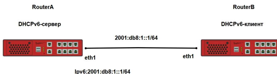
Рисунок 22 – Схема настройки встроенного сервера и клиента DHCPv6
