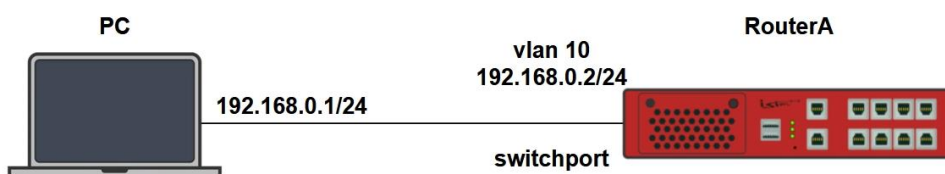
Рисунок 12 – Схема настройки работы L2 filter
