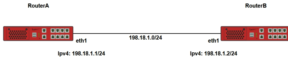
Рисунок 92 – Схема настройки межсетевого экранирования на основе номера порта (TCP/UDP) назначения
