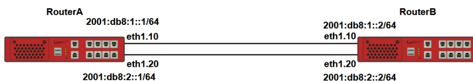
Рисунок 98 – Схема настройки работы ACL IPv6
