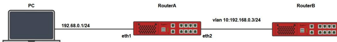
Рисунок 11 – Схема настройки L2 mangle list
