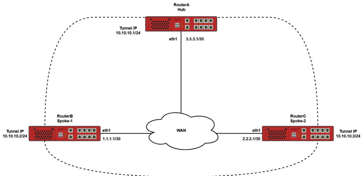
Рисунок 62 – Схема настройки DMVPN
