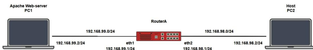
Рисунок 106 – Схема настройки Snort
