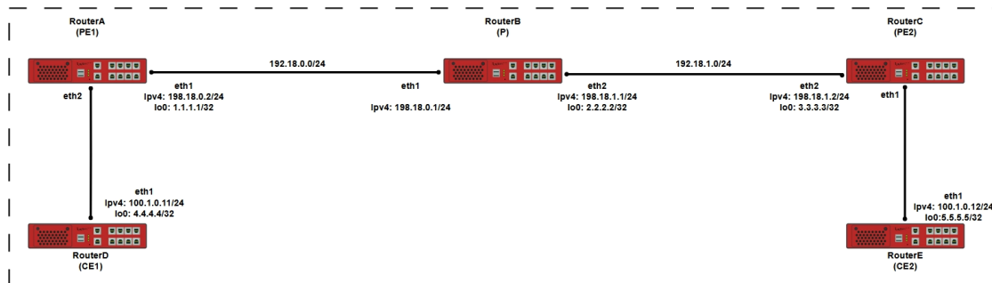
Рисунок 67 – Схема создания виртуальных частных сетей второго уровня (MPLS L2VPN) по технологиям VPLS
