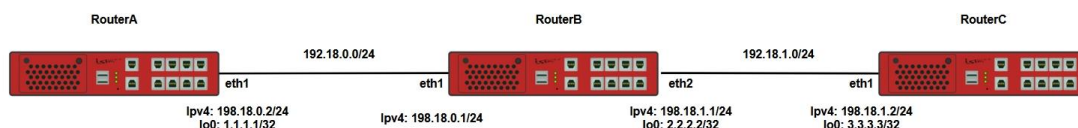
Рисунок 70 – Схема настройки виртуальных частных сетей второго уровня (MPLS L2VPN) по технологиям VPWS
