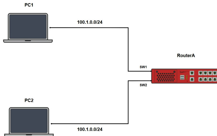
Рисунок 53 – Схема настройки Jumbo Frames
