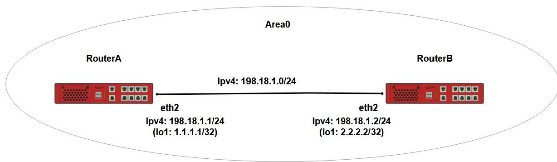
Рисунок 29 – Схема настройки динамической маршрутизации OSPFv2
