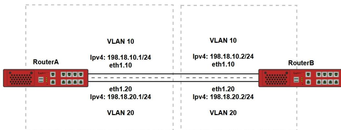
Рисунок 90 – Схема настройки межсетевого экранирования на основе IP-адреса назначения
