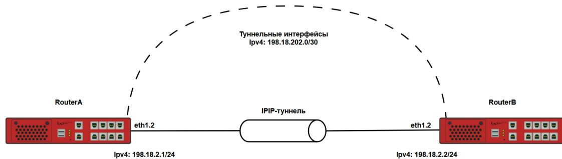
Рисунок 58 – IPIP-туннель
