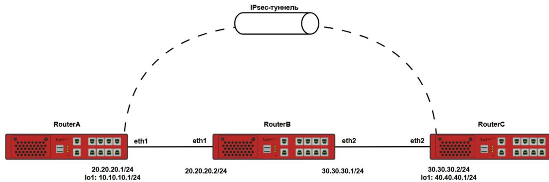
Рисунок 63 – Схема настройки протокола IPsec
