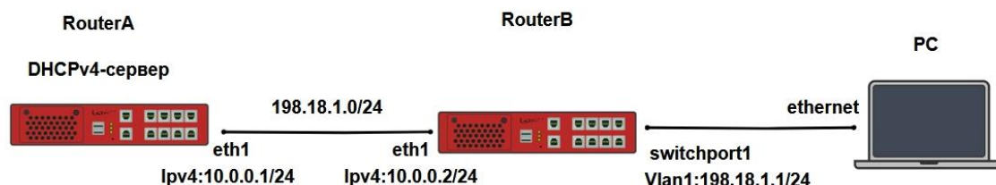
Рисунок 17 – Настройка DHCP Relay Option 82
