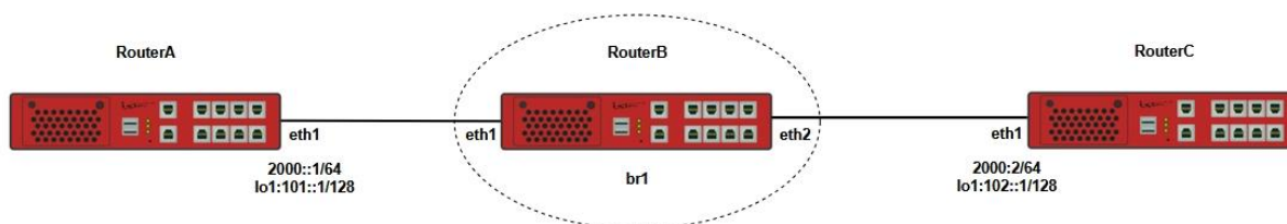
Рисунок 39 – Схема настройки протокола BFD IPv6 для статической маршрутизации
