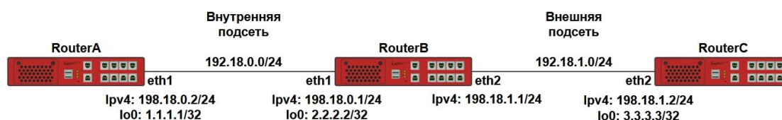
Рисунок 40 – Схема настройки Source NAT
