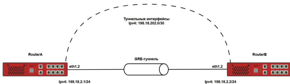
Рисунок 57 – GRE-туннель
