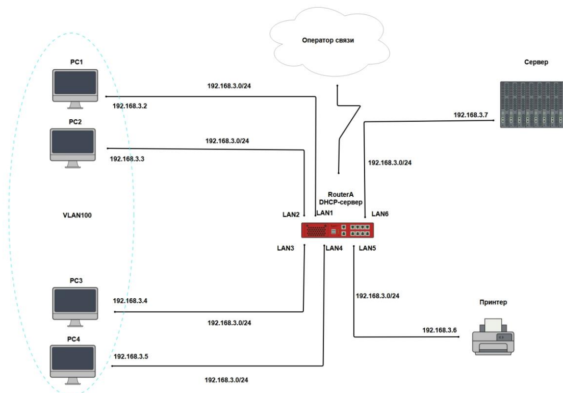
Рисунок 3 – Схема настройки локальной сети
