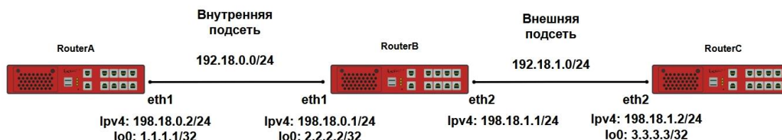
Рисунок 41 – Схема настройки Destination NAT
