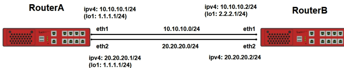
Рисунок 50 – Вариант назначения в качестве next-hop для статического маршрута двух интерфейсов
