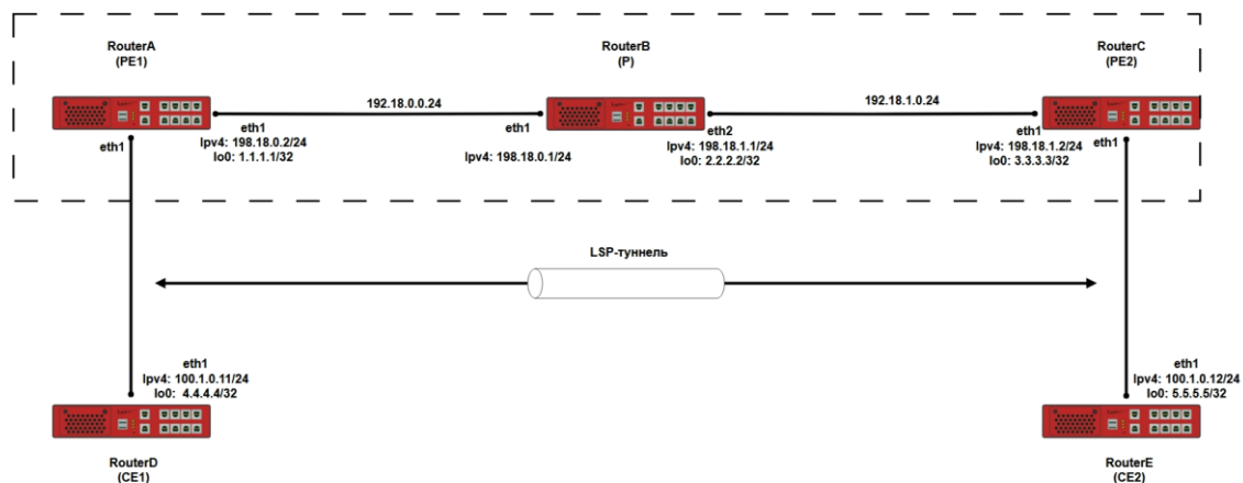
Рисунок 66 – Схема настройки виртуальных частных сетей второго уровня (MPLS L2VPN) по технологиям VPWS
