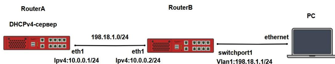
Рисунок 18 – Схема настройки DHCP Relay
