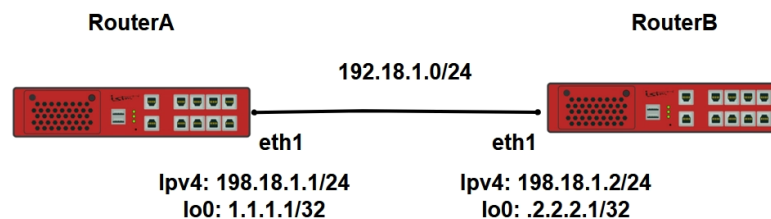
Рисунок 49 – Схема настройки физического интерфейса в качестве next-hop
