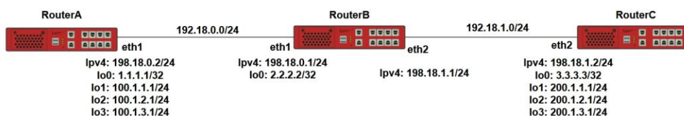
Рисунок 34 – Схема настройки фильтрации маршрутов с помощью prefix-list
