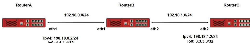
Рисунок 38 – Схема настройки протокола BFD
