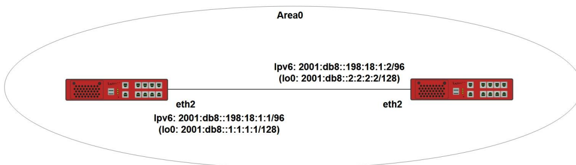
Рисунок 30 – Схема настройки динамической маршрутизации OSPFv3
