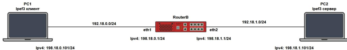
Рисунок 78 – Настройка предотвращения перегрузки очередей RED
