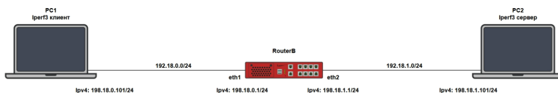
Рисунок 83 – Схема настройки
