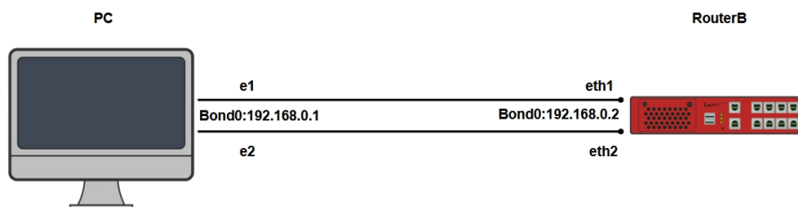
Рисунок 85 – Схема настройки протокола Bond
