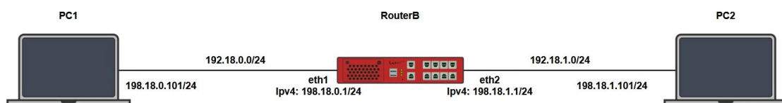
Рисунок 75 – Настройка работы QoS дисциплины обслуживания CBQ
