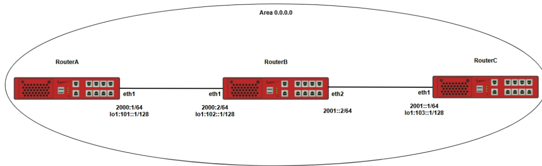
Рисунок 37 – Схема настройки протокола BFD IPv6 для динамической маршрутизации
