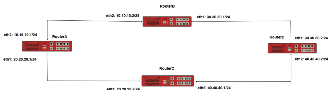
Рисунок 113 – Схема настройки IP SLA
