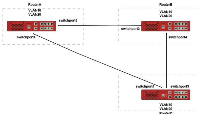
Рисунок 9 – Схема настройки протокола MSTP
