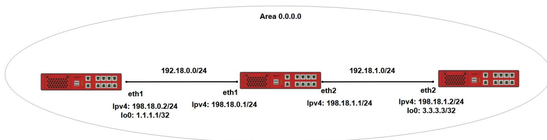
Рисунок 36 – Схема настройки протокола BFD для динамической маршрутизации
