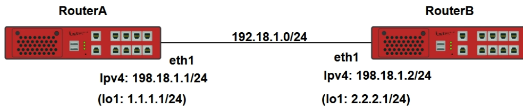
Рисунок 25 – Схема настройки статической маршрутизации
