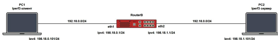
Рисунок 79 – Настройка предотвращения перегрузки очередей GRED
