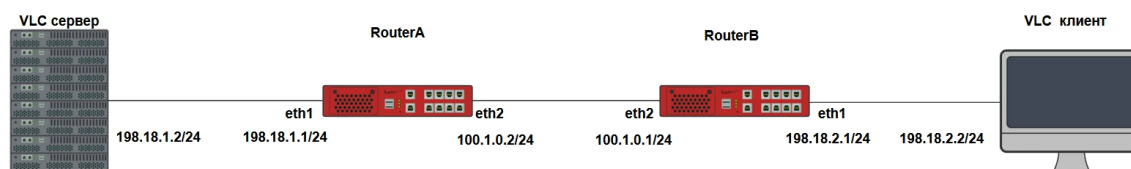
Рисунок 71 – Схема настройки PIM и IGMP
