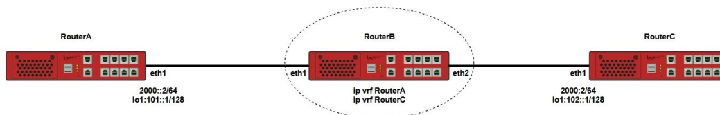
Рисунок 44 – Схема настройки VRF Lite Ipv6
