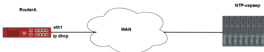
Рисунок 109 – Схема настройки NAT masquerade
