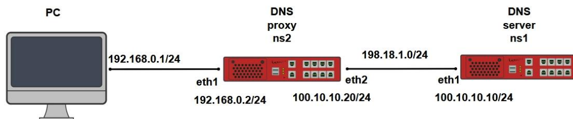
Рисунок 19 – Схема настройки DNS proxy
