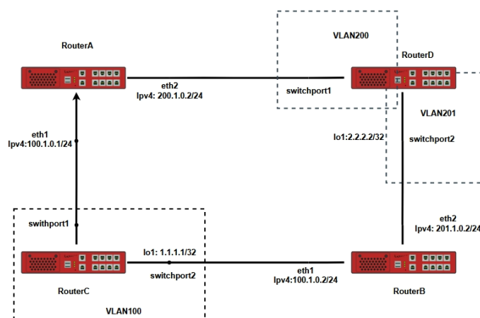
Рисунок 86 – Схема настройки протокола CARP
