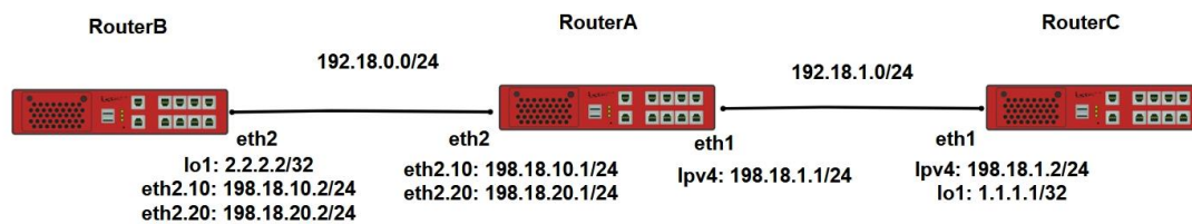
Рисунок 47 – Схема настройки PBR на основе номера порта источника
