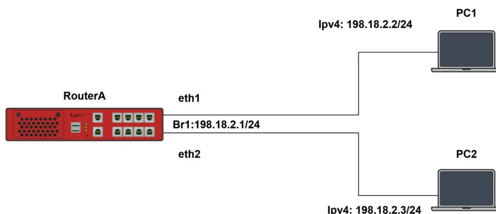
Рисунок 4 – Схема настройки моста
