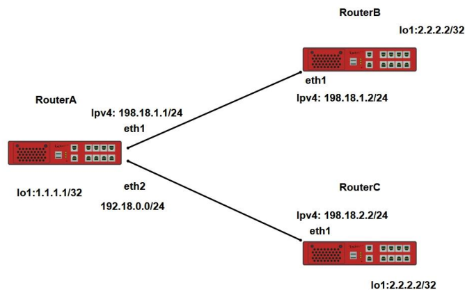
Рисунок 46 – Схема настройки PBR на основе IP-адреса назначения
