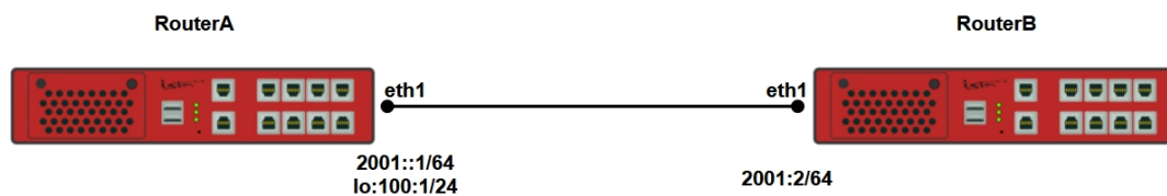
Рисунок 56 – Схема настройки протокола PPPoE IPv6
