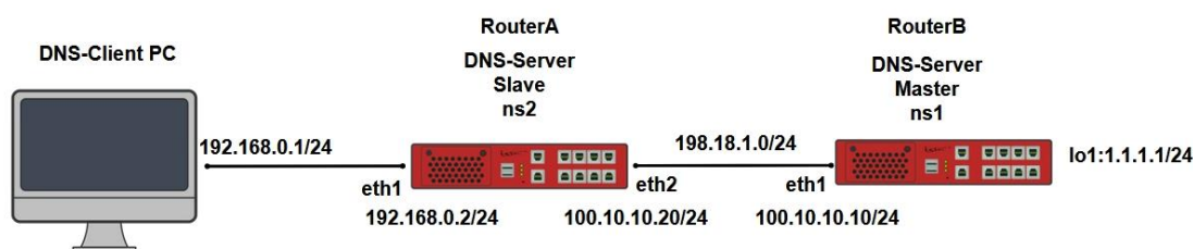
Рисунок 20 – Схема настройки DNS server
