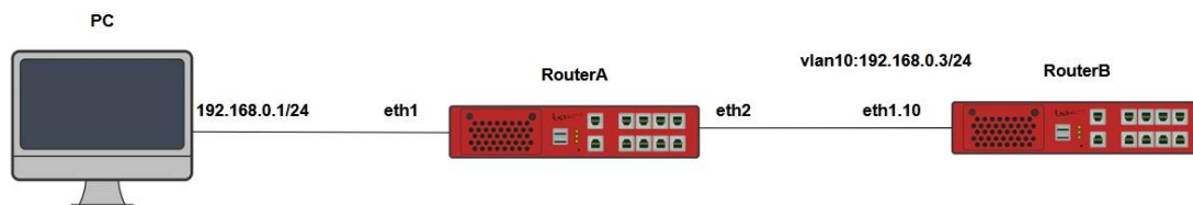
Рисунок 10 – Схема настройки L2 ACL
