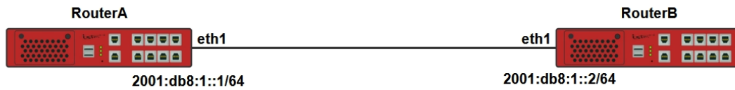
Рисунок 100 – Схема настройки межсетевого экранирования на основе номера порта (TCP/UDP) источника (IPv6)
