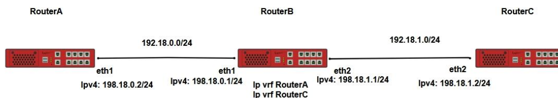
Рисунок 43 – Схема настройки VRF Lite
