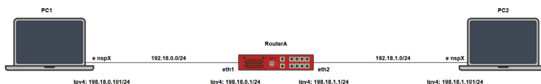
Рисунок 82 – Схема настройки дисциплины WRED
