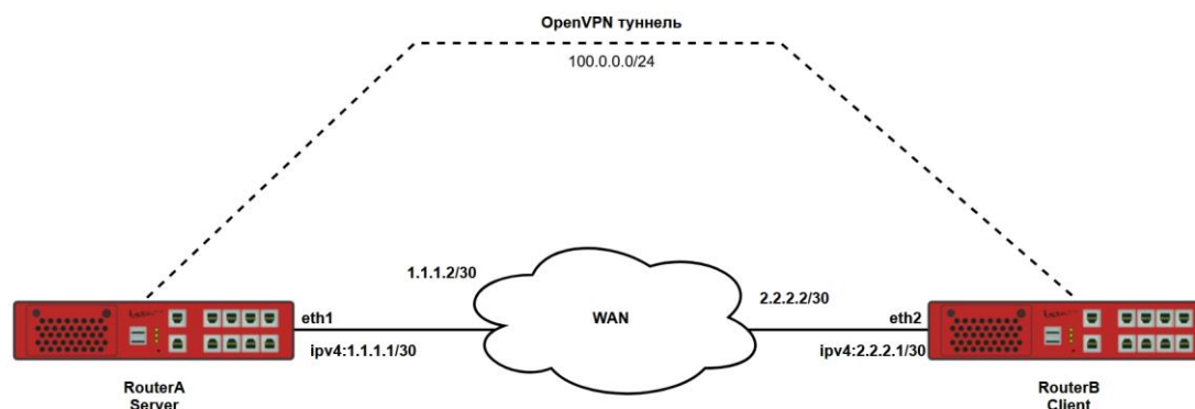
Рисунок 61 – Схема настройки OpenVPN
