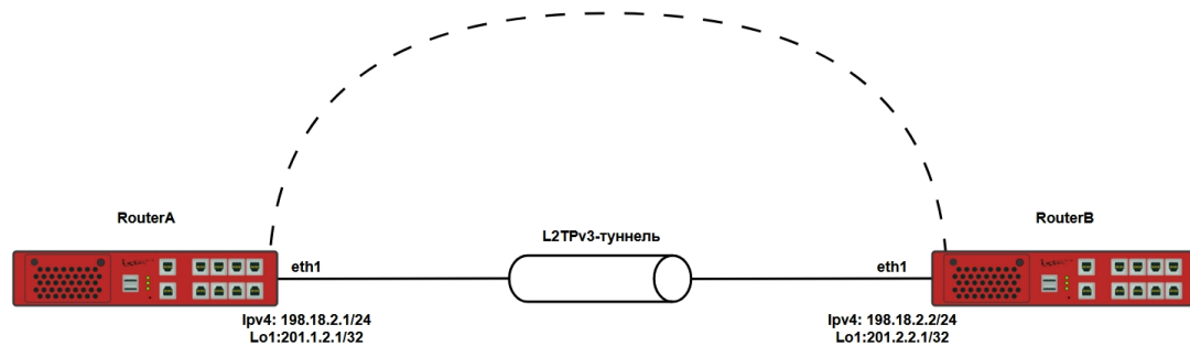
Рисунок 60 – L2TPv3-туннель
