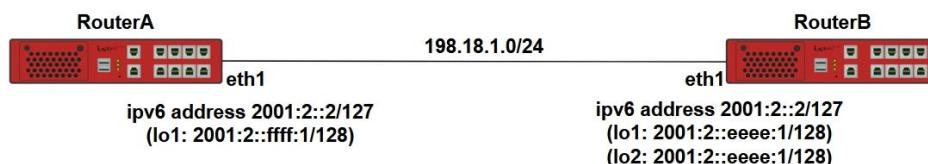
Рисунок 28 – Схема настройка протокола динамической маршрутизации RIPng
