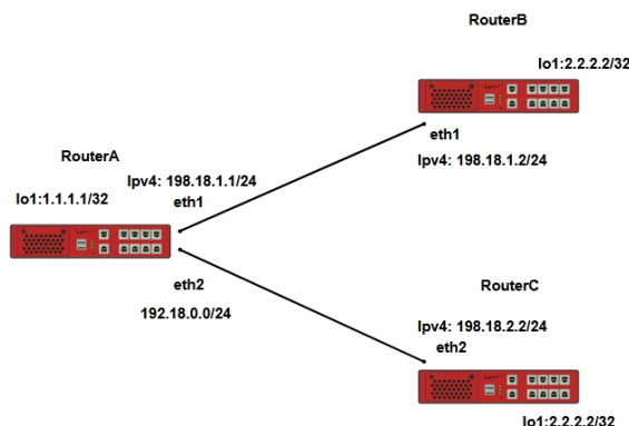
Рисунок 45 – Схема настройки PBR на основе IP-адреса источника
