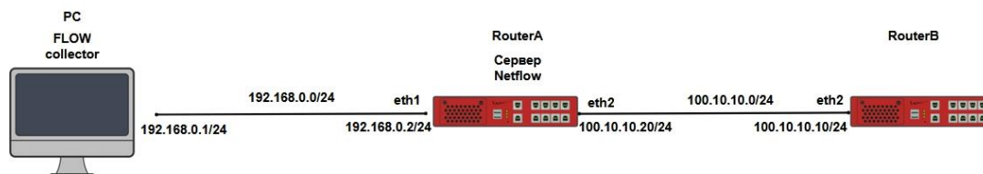
Рисунок 110 – Схема настройки утилиты мониторинга Netflow
