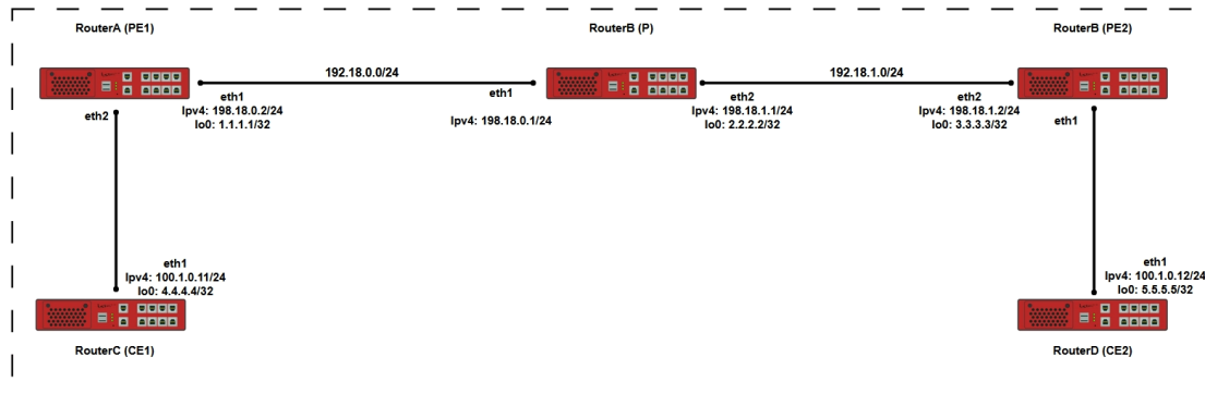
Рисунок 69 – Схема настройки виртуальных частных сетей второго уровня (MPLS L2VPN) по технологиям VPLS с BGP сигнализацией
