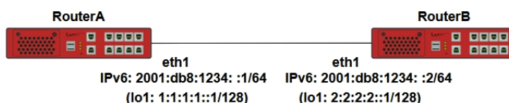
Рисунок 26 – Схема настройки статической маршрутизации IPv6
