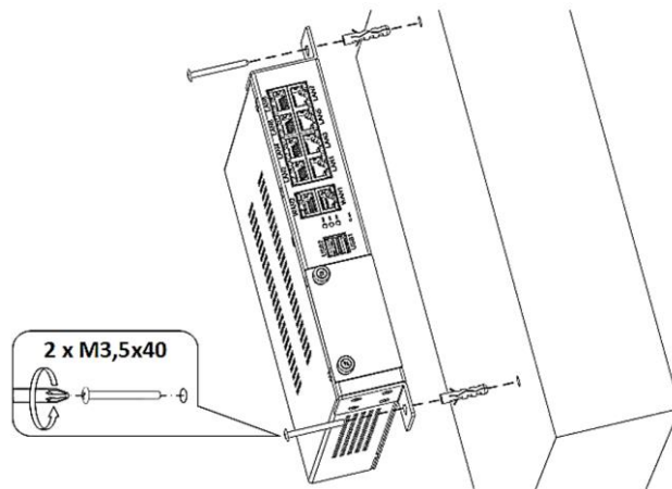
Рисунок 58 – Крепление изделий к стене с использованием комплекта КРПГ.465961.002
