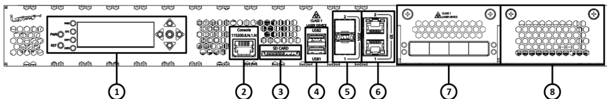
Рисунок 36 – Конфигурация элементов передней панели изделия ISN50502T5-M16A
