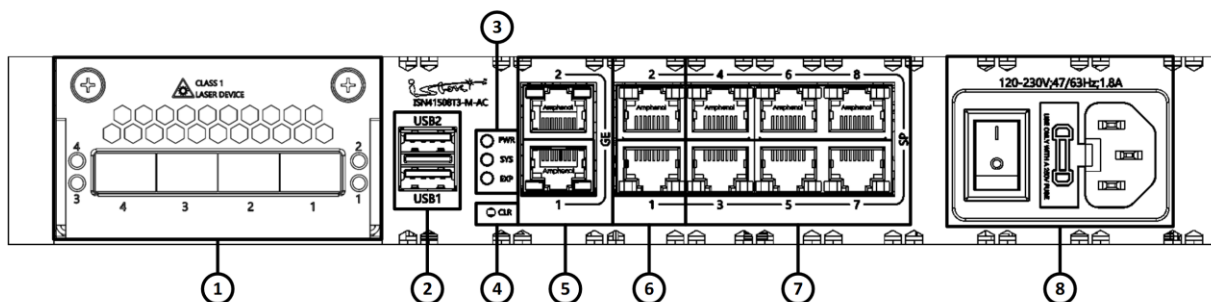
Рисунок 20 – Конфигурация элементов передней панели изделия ISN41508T3-M-AC/ISES0108
