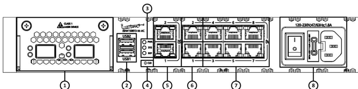
Рисунок 18 – Конфигурация элементов передней панели изделия ISN41508T3-M-AC/ISES1004
