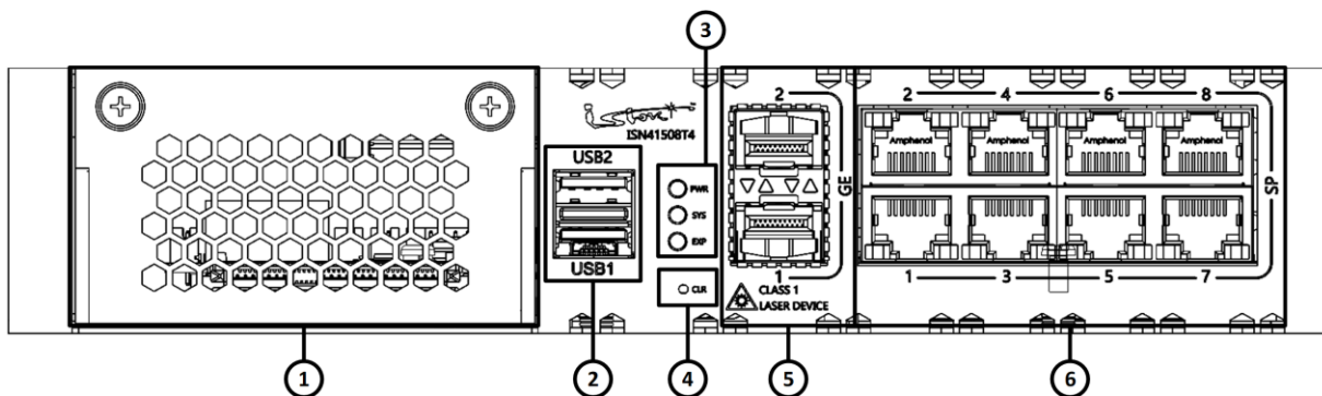
Рисунок 7 – Конфигурация элементов передней панели изделия ISN41508T4
