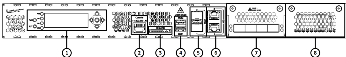
Рисунок 28 – Конфигурация элементов передней панели изделия ISN50502T5-M12A
