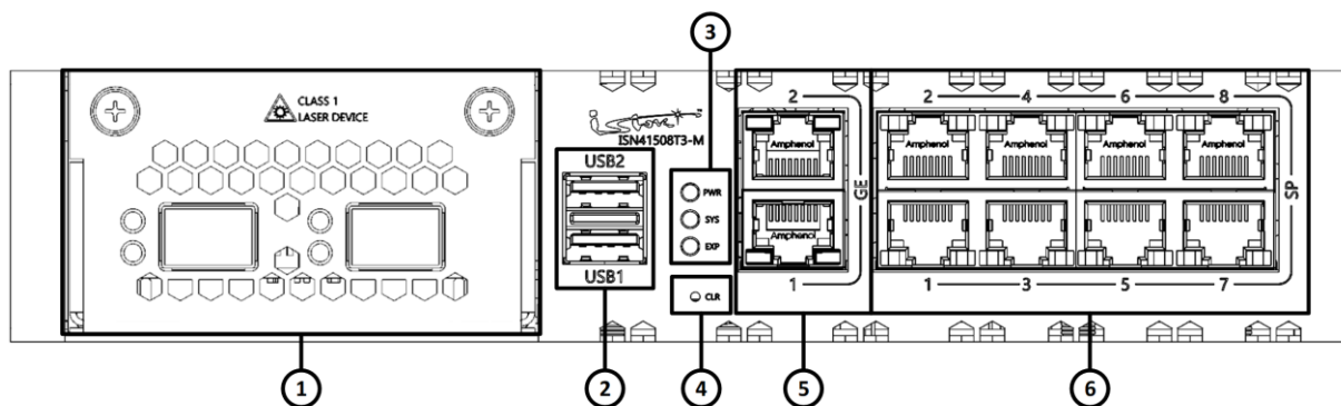
Рисунок 12 – Конфигурация элементов передней панели изделия ISN41508T3-M/ISES1004
