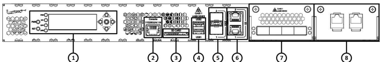
Рисунок 30 – Конфигурация элементов передней панели изделия ISN50502T5-M13A
