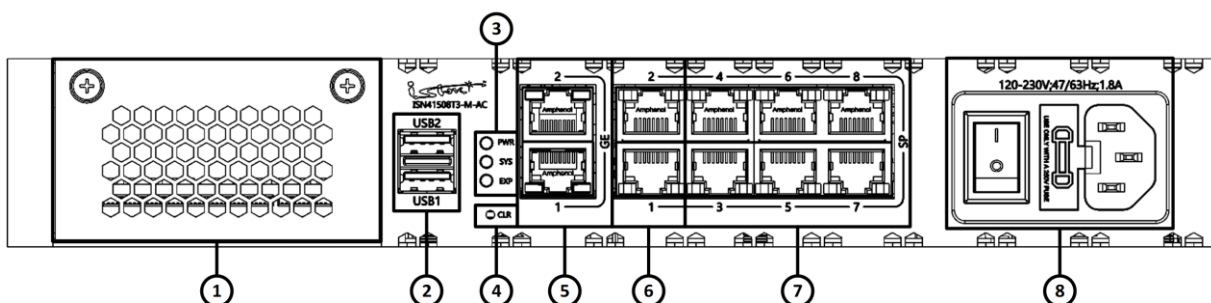
Рисунок 9 – Конфигурация элементов передней панели изделия ISN41508T3-M-AC
