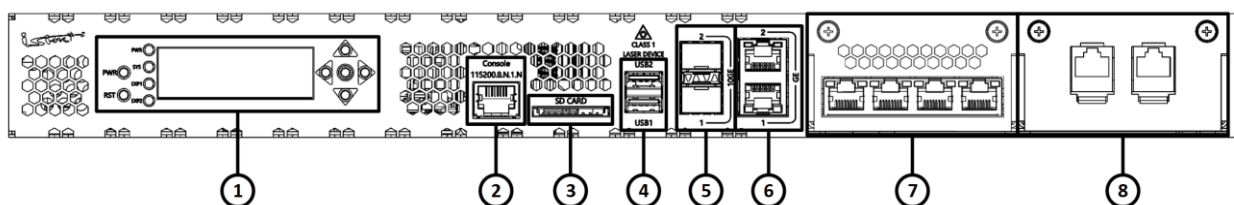
Рисунок 26 – Конфигурация элементов передней панели изделия ISN50502T5-M11A
