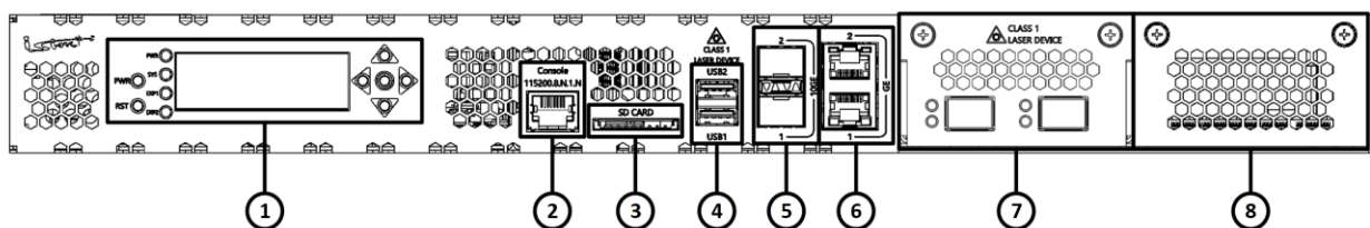
Рисунок 34 – Конфигурация элементов передней панели изделия ISN50502T5-M15A
