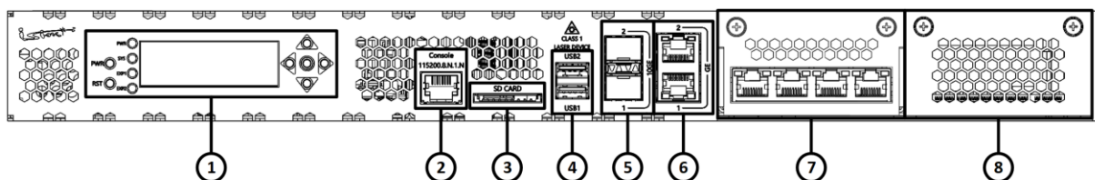
Рисунок 24 – Конфигурация элементов передней панели изделия ISN50502T5-M10A
