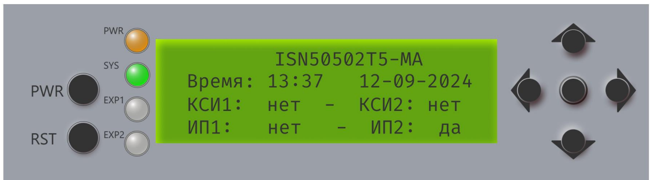
Рисунок 1.22 – Пример стартового экрана при отказе первого блока питания
