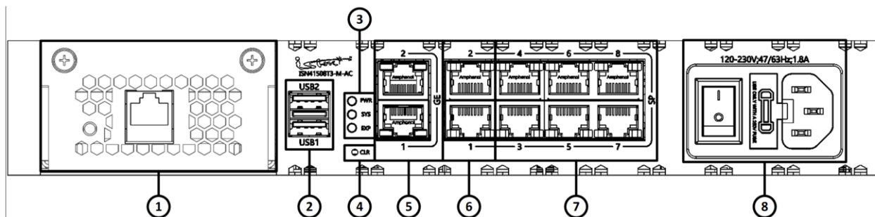
Рисунок 45 – Конфигурация элементов передней панели изделия
