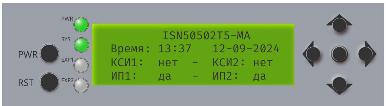
Рисунок 1.4 – Пример состояния дисплея и индикаторов после включения платформы кнопкой PWR
