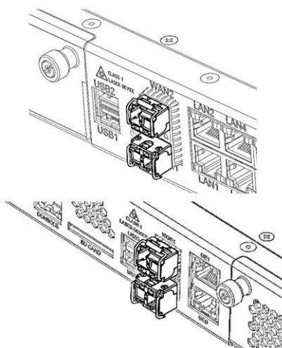
Рисунок 59 – SFP-трансиверы, установленные в слоты изделия
