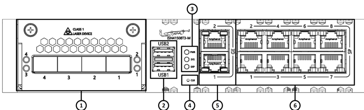
Рисунок 14 – Конфигурация элементов передней панели изделия ISN41508T3-M/ISES0108
