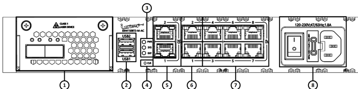
Рисунок 22 – Конфигурация элементов передней панели изделия ISN41508T3-M-AC/ISES0116
