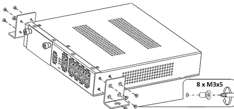
Рисунок 57 – Крепление уголков из комплекта КРПГ.465961.002
