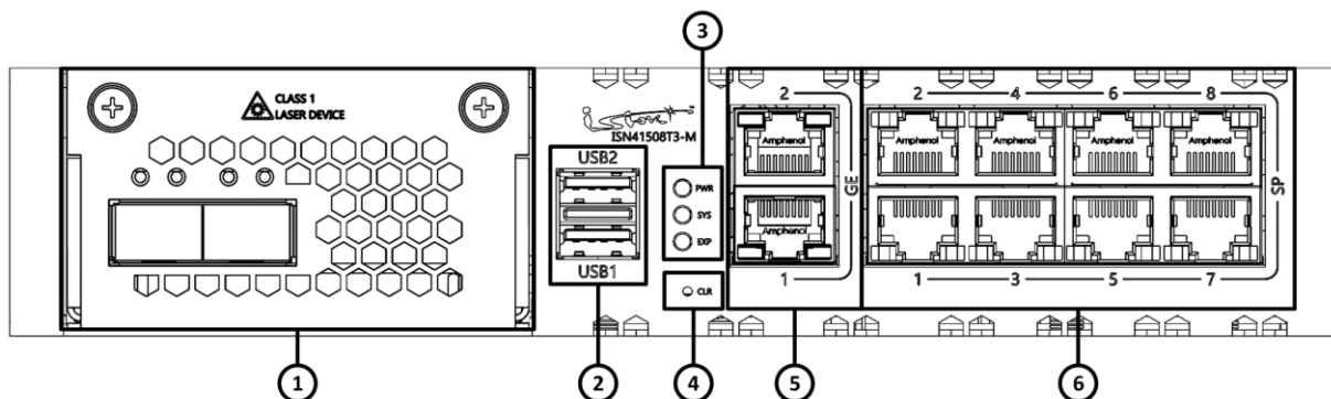
Рисунок 16 – Конфигурация элементов передней панели изделия ISN41508T3-M/ISES0116
