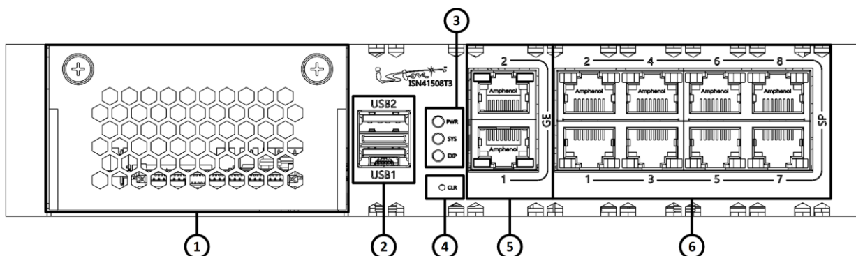
Рисунок 2 – Конфигурация элементов передней панели изделия ISN41508T3
