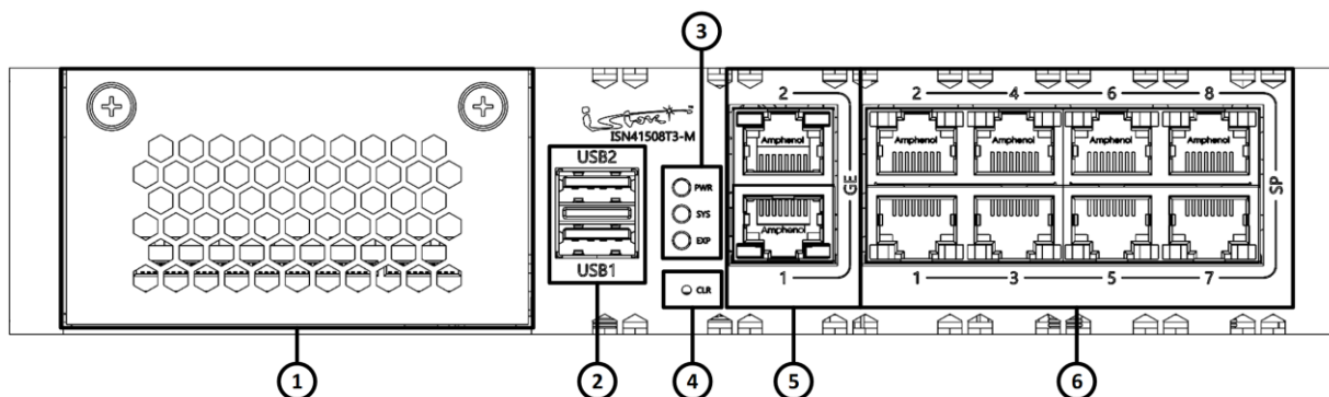
Рисунок 5 – Конфигурация элементов задней панели изделия ISN41508T3-M
