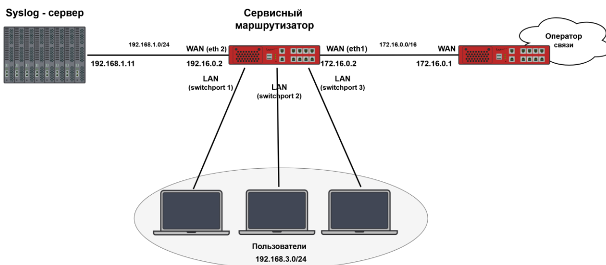
Рисунок 20 – Схема настройки журналирования событий на удаленный Syslog-сервер
