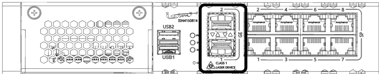
Рисунок 6 – WAN-порты. Передняя панель ISN41508T4
