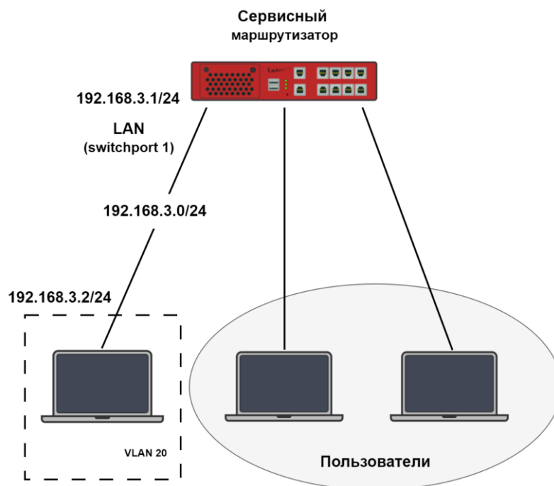
Рисунок 15 – Схема настройки локальной сети
